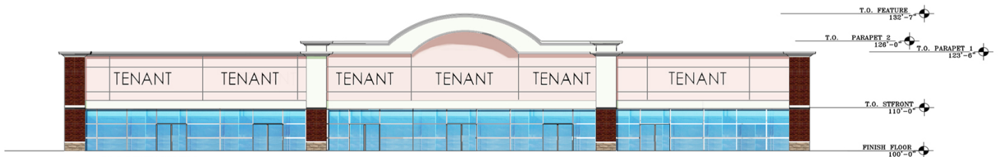
Proposed Elevation SCALE: N.T.S.
