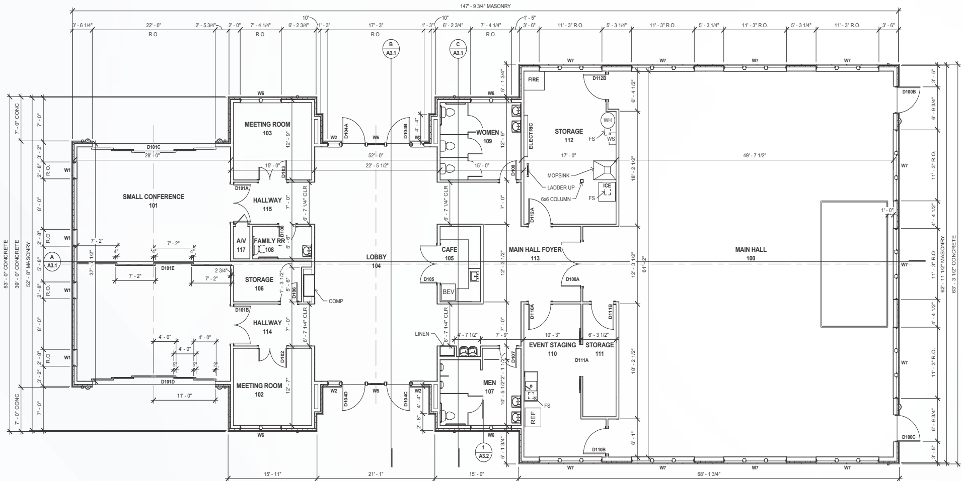
A FLOOR PLAN SCALE: 1/8" = 1'-0"
