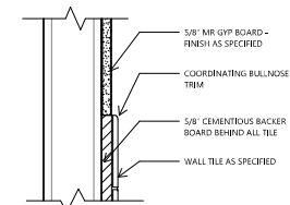
5 TILE EDGE TRANSITION
