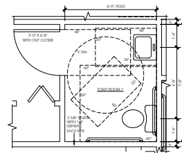
TOILET ROOM 1
