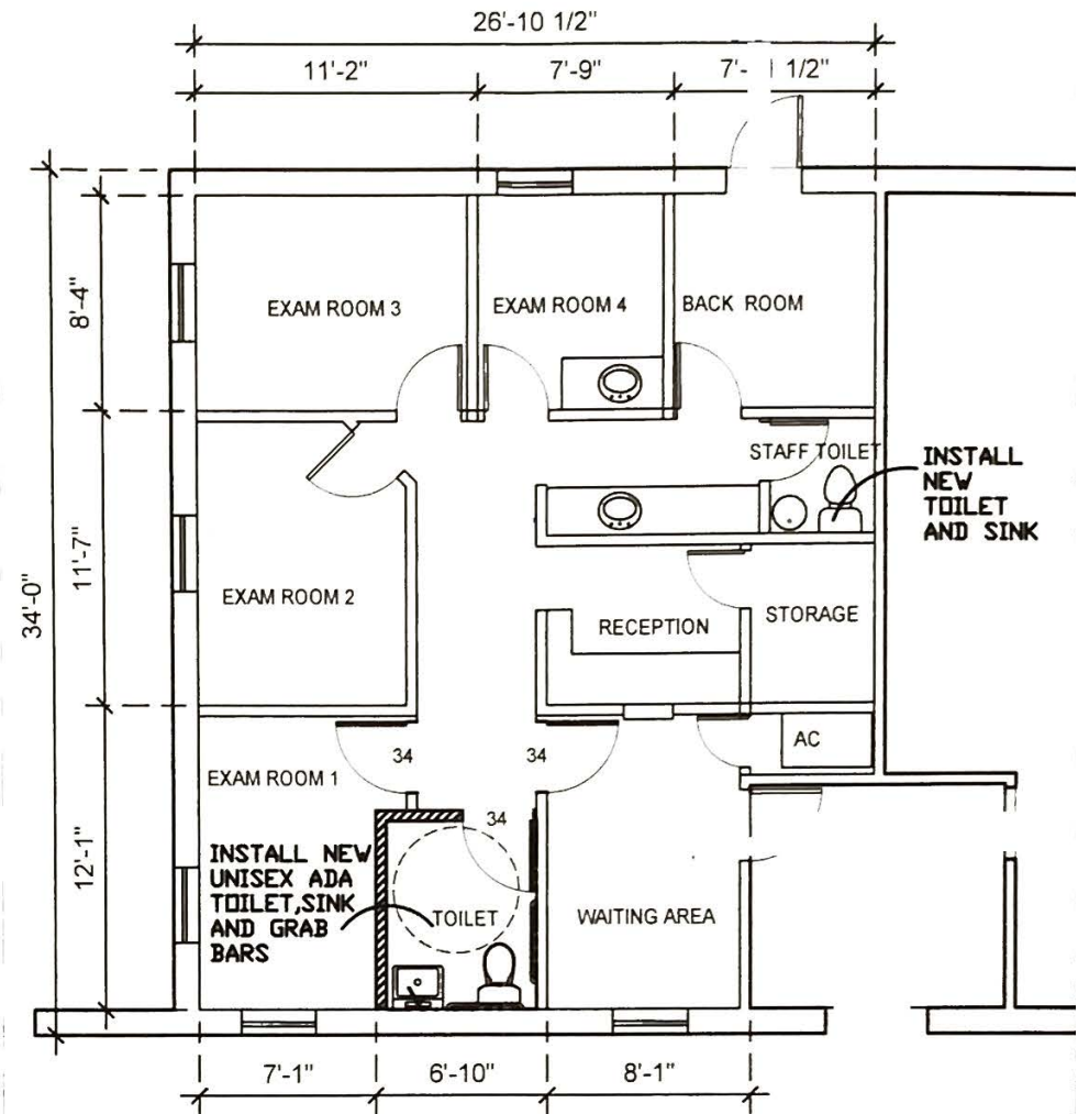
02 SUITE A-FLOOR PLAN 1/8" : 1'-0" 890 SF
