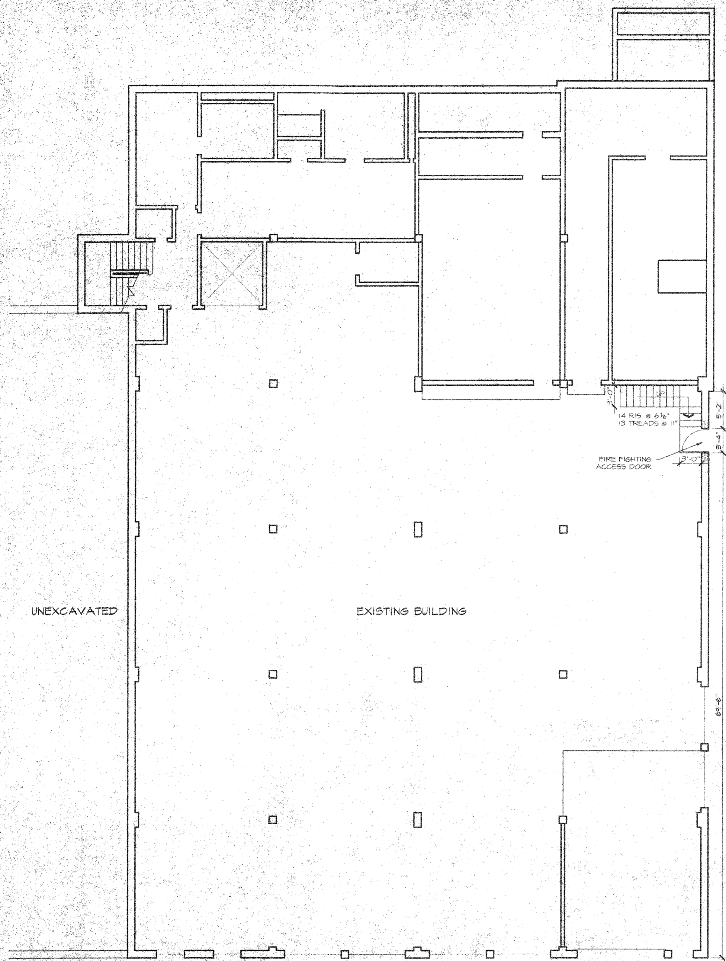
LOWER LEVEL PLAN SCALE: 1/8" = 1'-0"
