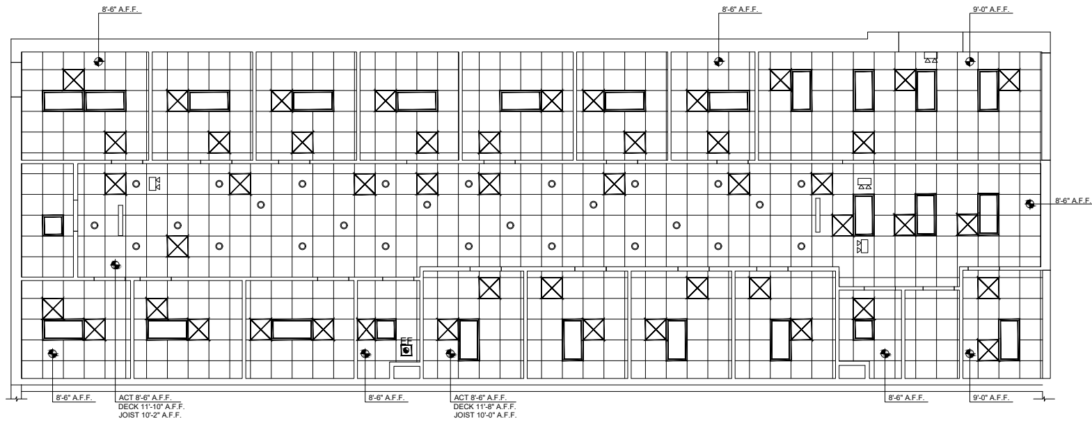
REFLECTED CEILING PLAN N.T.S.
