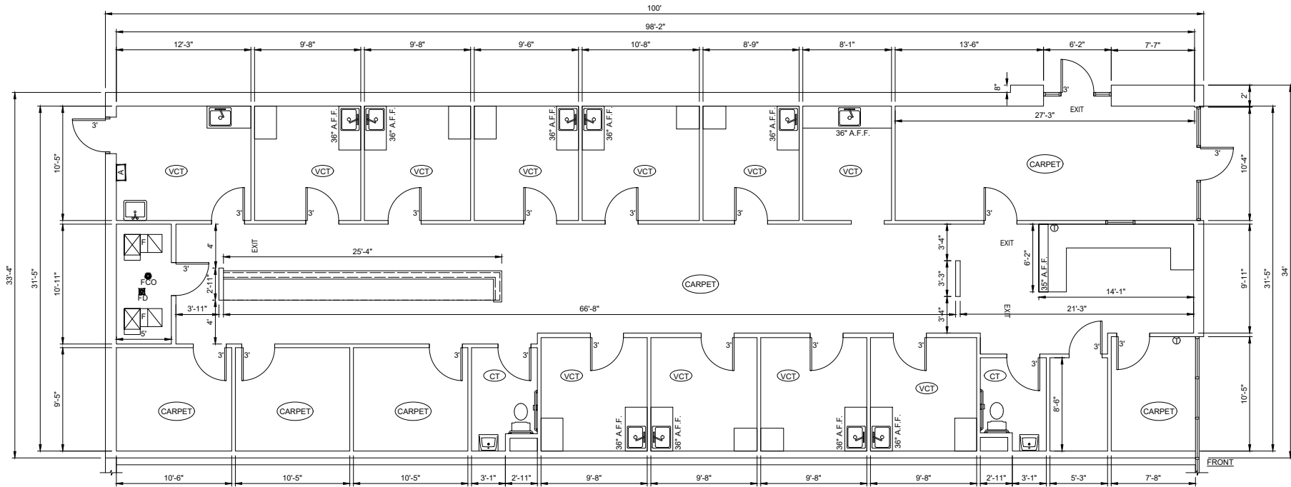
FLOOR PLAN N.T.S.
