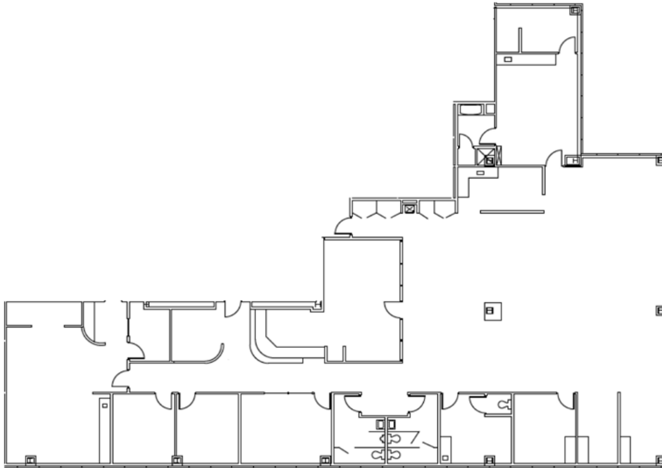
SUITE 5304 - 6,009 SF
