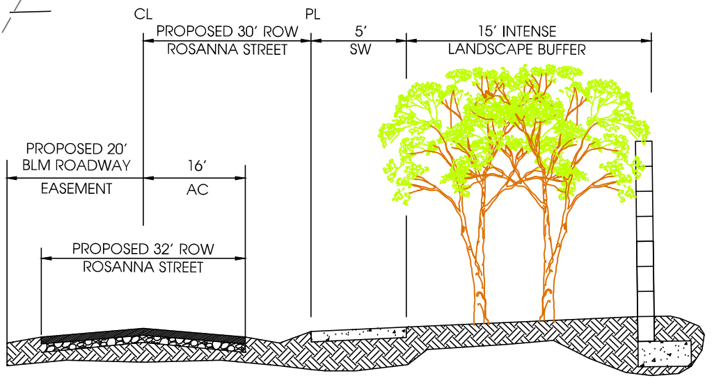
SECTION A SCALE: HORIZ 1" = 40'
