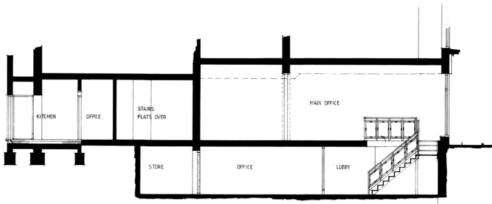
LONGITUDINAL SECTION
