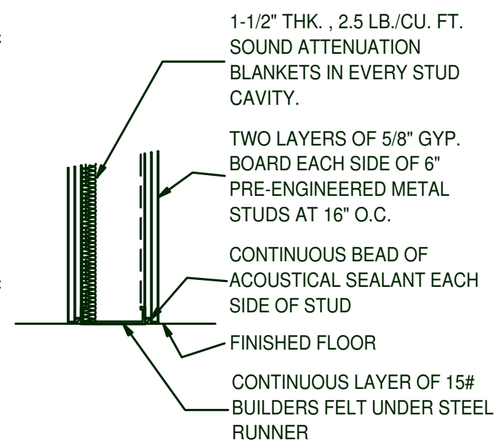
SECTION 1-A5 1" = 1' 0"
