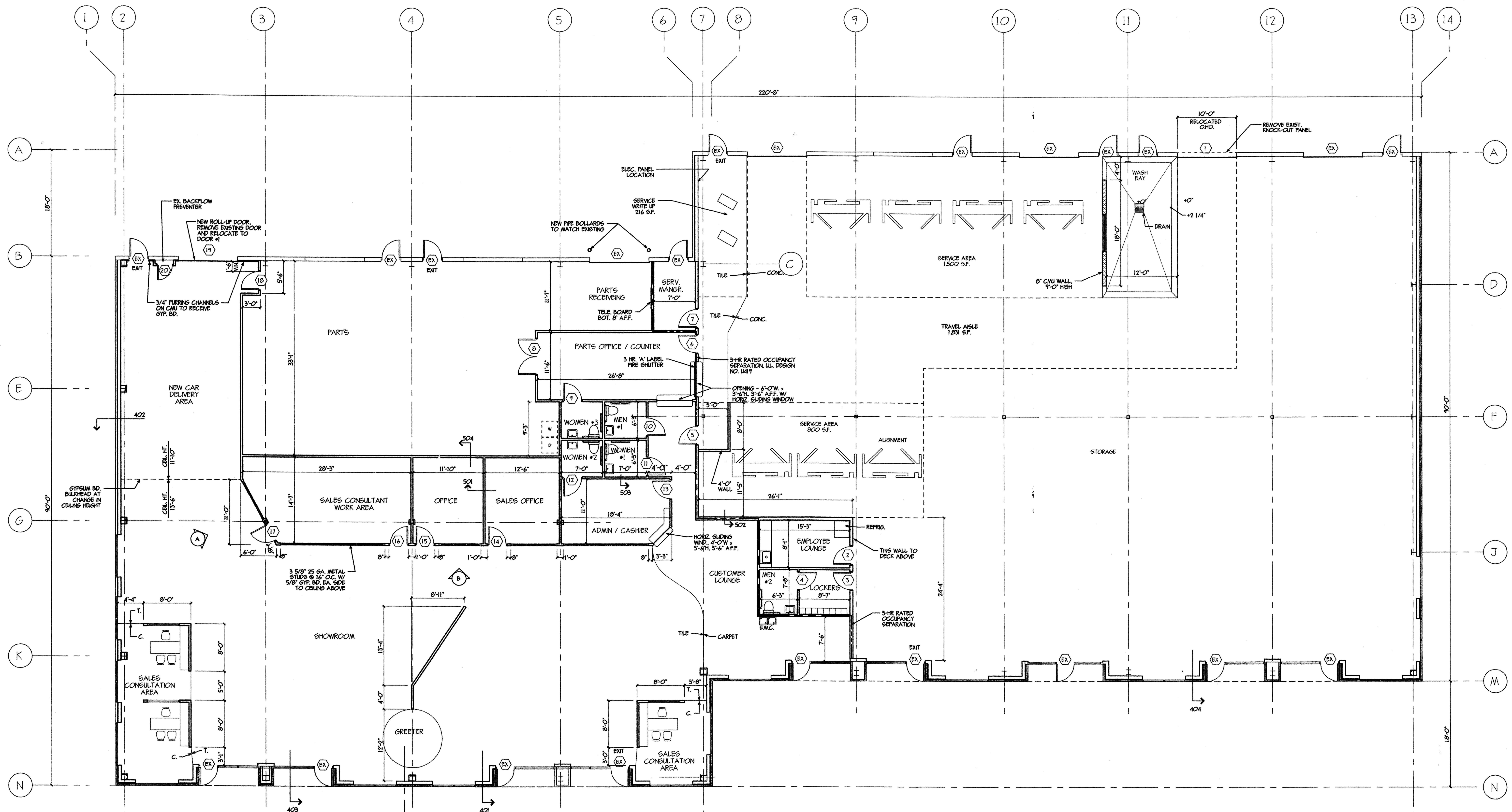
101 FLOOR PLAN SCALE: 1/8" = 1'-0"
