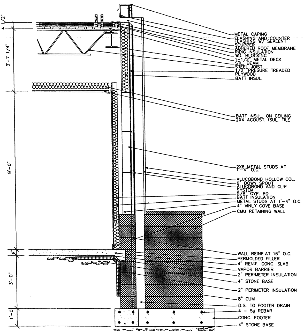
SECTION B-B SCALE: 3/4" = 1'-0"
