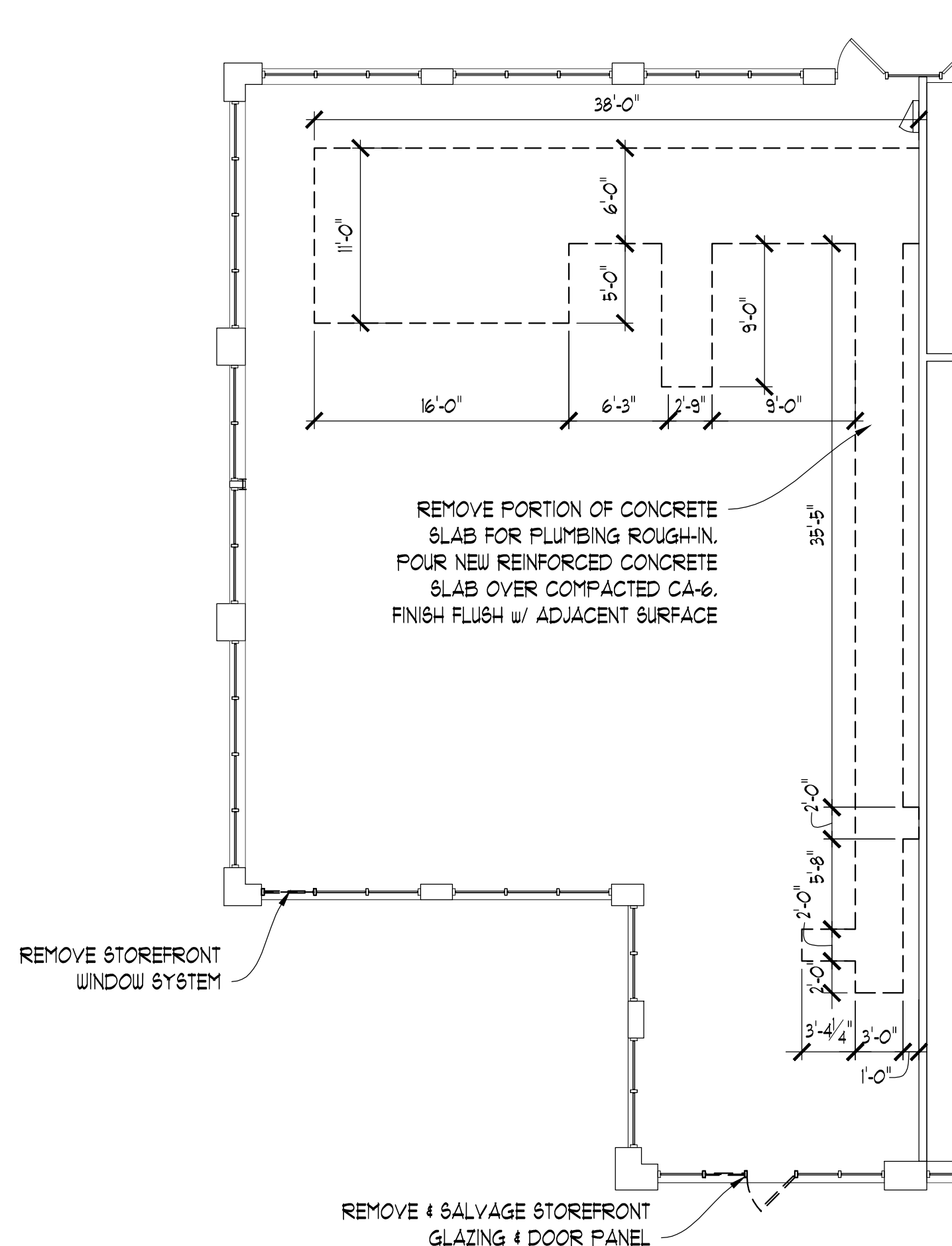
DEMOLITION PLAN SCALE: 1/8" = 1'-0"
