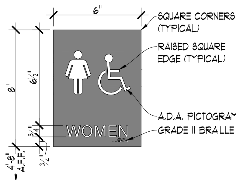
3 RESTROOM SIGNAGE DETAIL SCALE: N.T.S.
