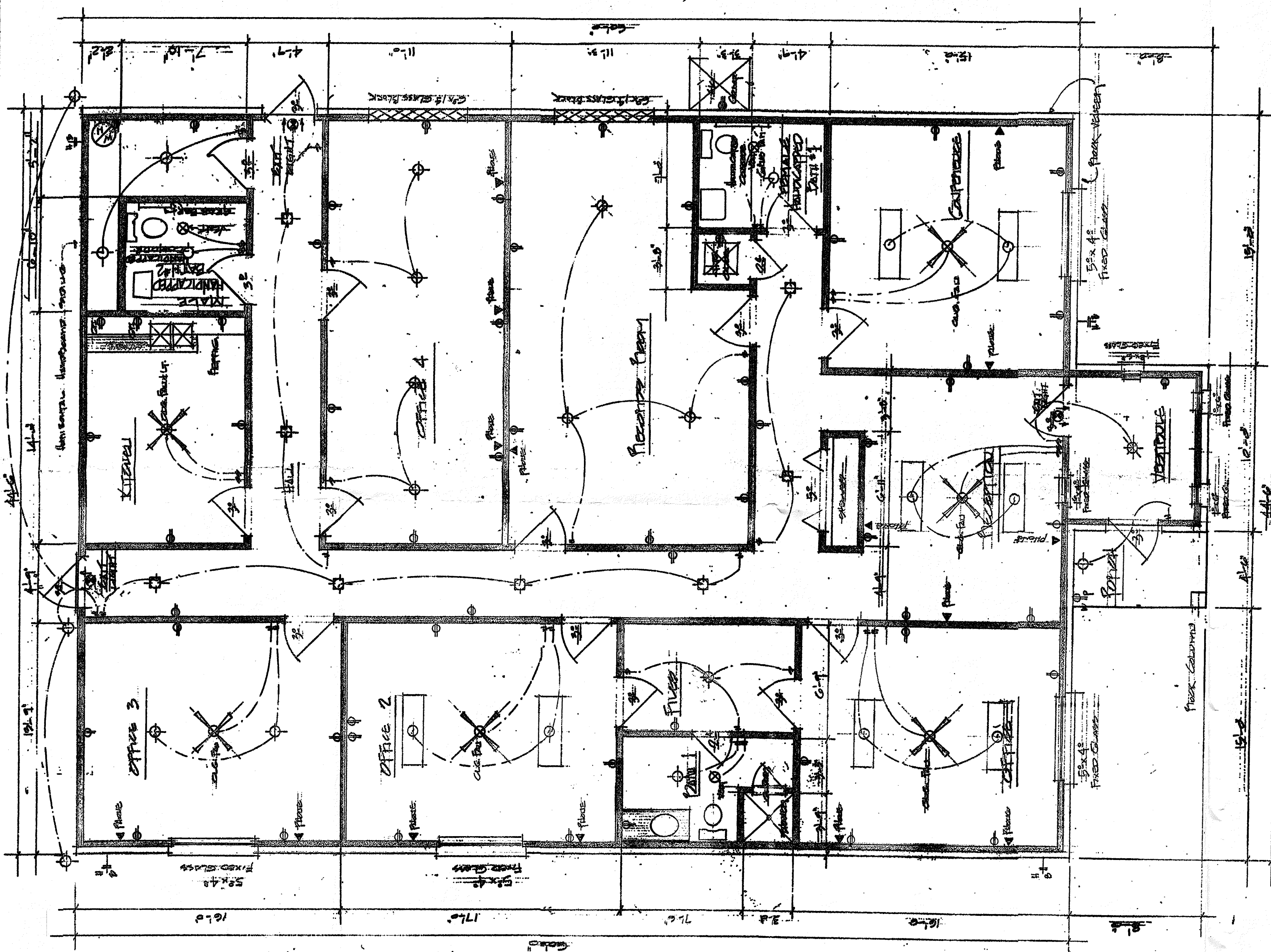
F L O O R P L A N 1/4" = 1'-0"
