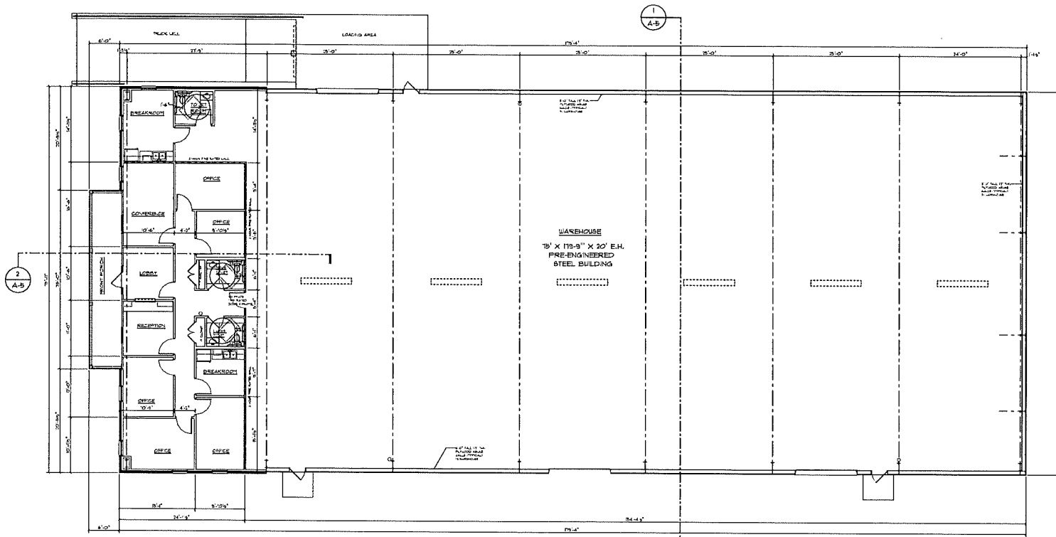
1 FLOOR PLAN SCALE: 1/8" = 1'-0"
