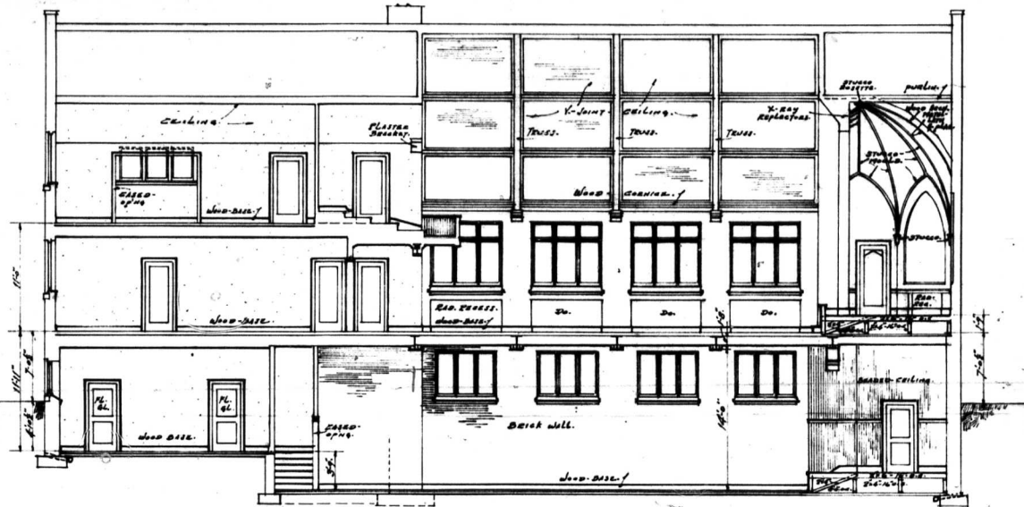
LONGITUDINAL SECTION. 1/8" scale.
