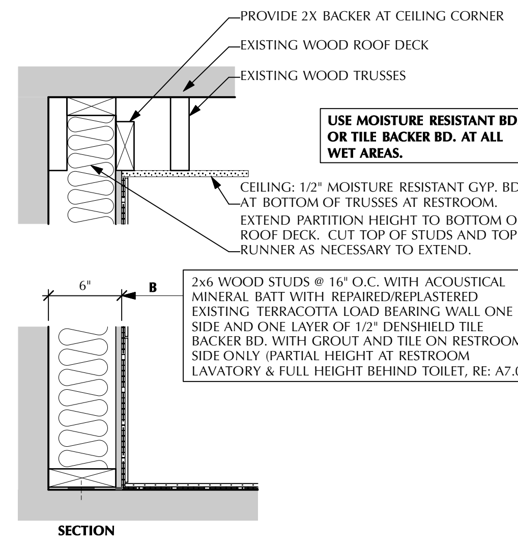
06 Partition Type B Scale: NTS
