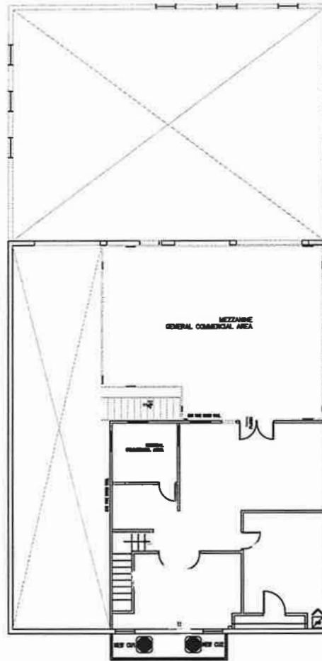
MEZZANINE PLAN SCALE: 1/8" = 1'-0"
